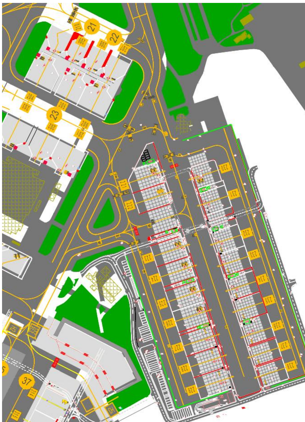
Figura 5. Pista 16L/34R - Arrivi piazzali 200
