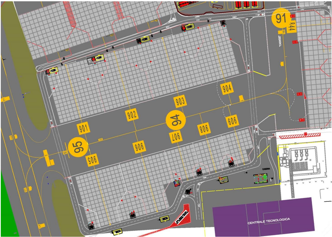
Figura 13. Pista 16L/34R - Arrivi piazzali 900
