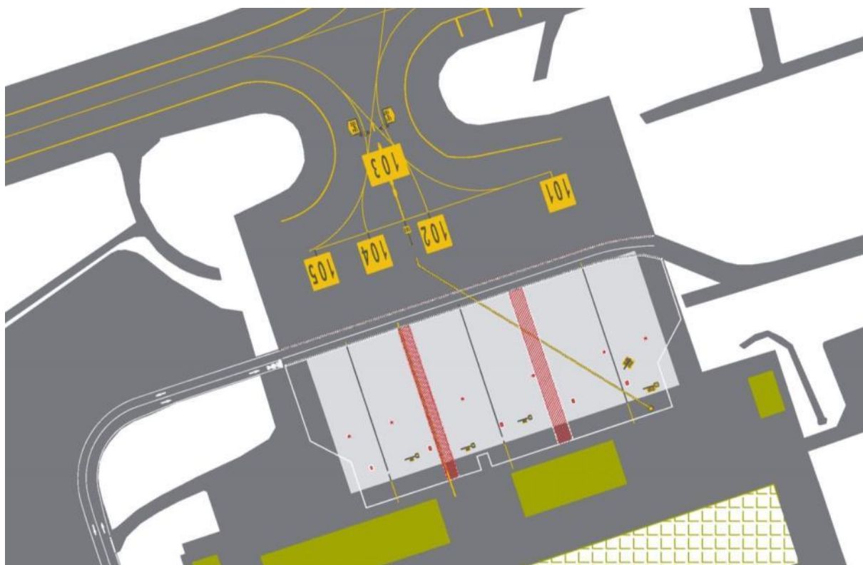
Figura 4. Pista 16L/34R - Arrivi piazzali serie 100
